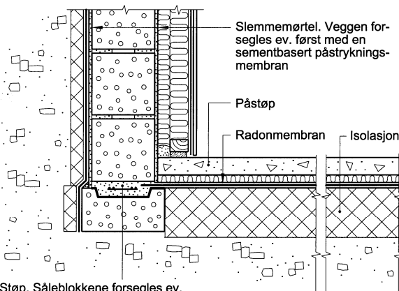
Fig. 2 Eksempel på bruk i bruksgruppe B Golv på grunnen og murt yttervegg mot terreng.
