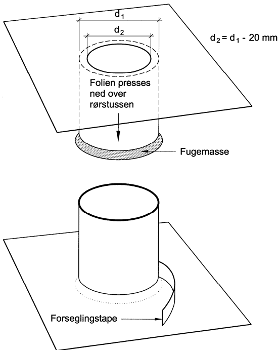
Fig. 8 Prinsipp for tetting rundt rørgjennomføringer Det lages hull i membranen som er litt mindre enn røret, og membranen presse over gjennomføringen etter at det først er plassert en fugemasse rundt røret. Fugen sikres med forseglingstape til slutt.
