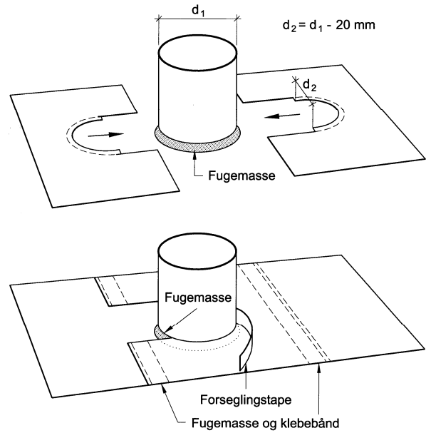
Fig. 9 Prinsipp for tetting rundt runde gjennomføringer der membranen ikke kan trekkes over gjennomføringen.
