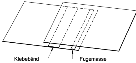
Fig. 6 Blackline 1000 Radonsperre skjøtes med klebebånd og fugemasse (alternativt kan disse plasseres motsatt).
